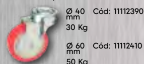
Rueda poliuretano pasante
