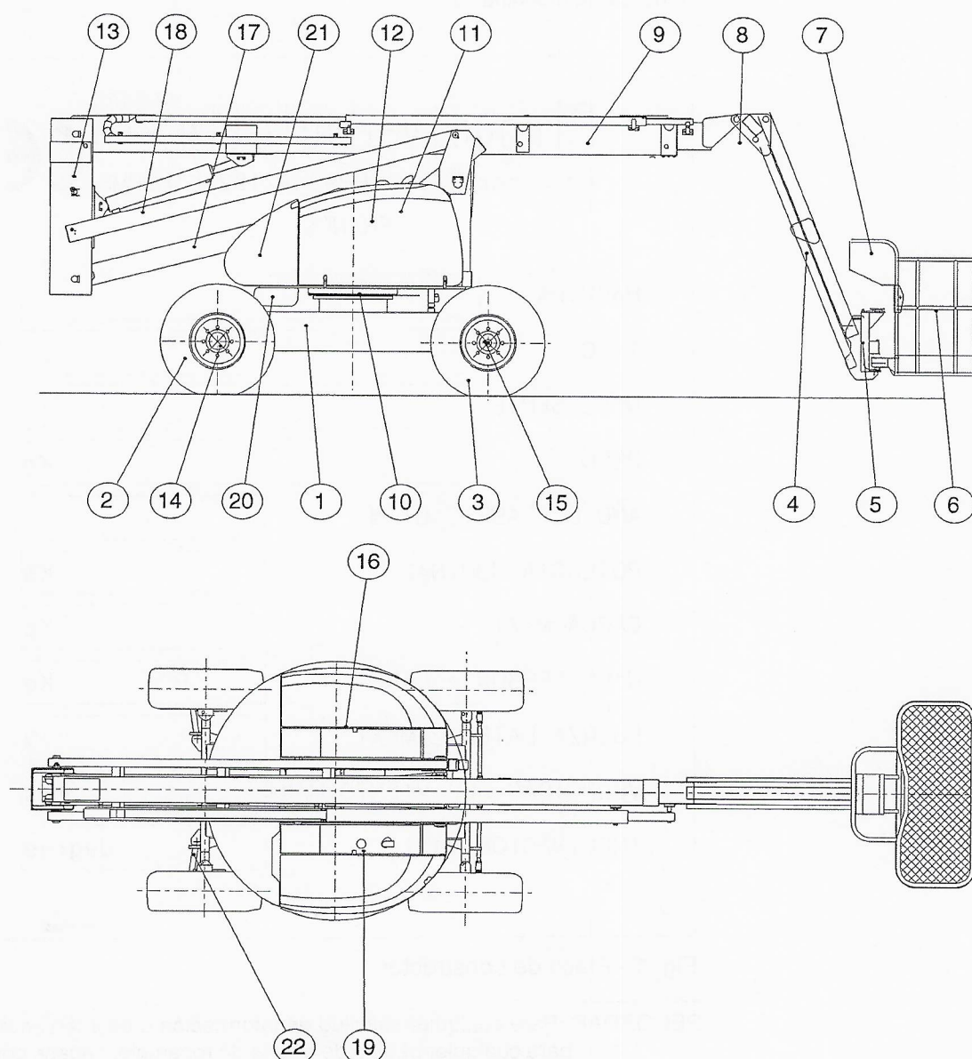
Fig. 2 - Localización principales componentes
