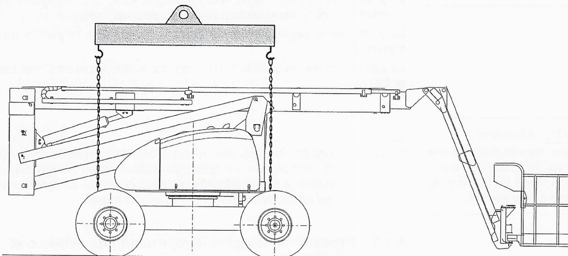
Fig. 3 - Descarga por elevación
