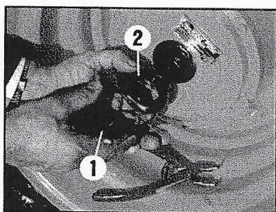
Fotografía 8 Desenganche
