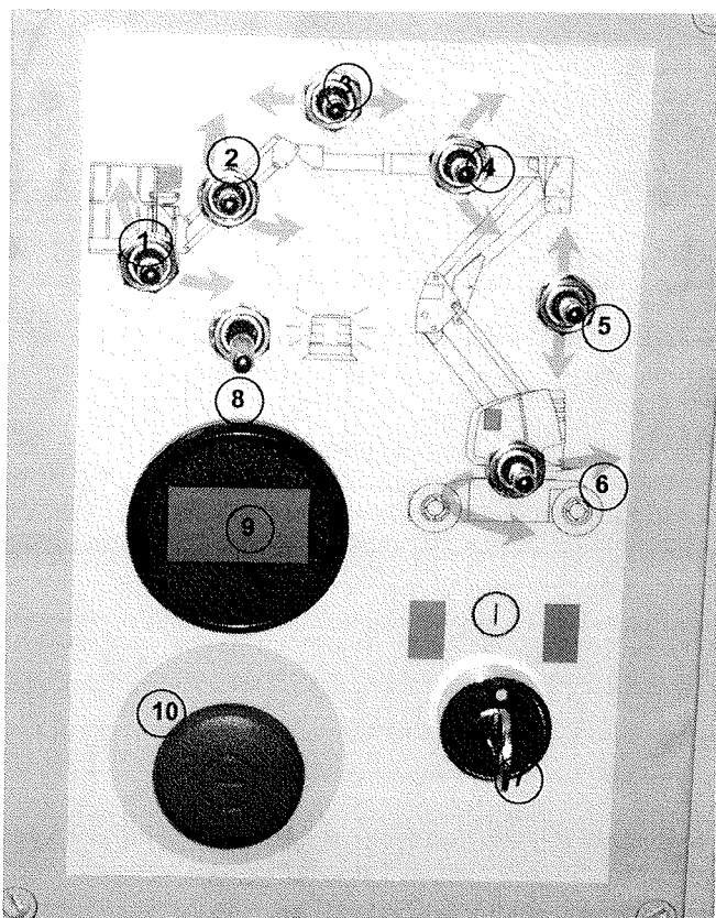
Foto 2: Puesto de mando torreta
