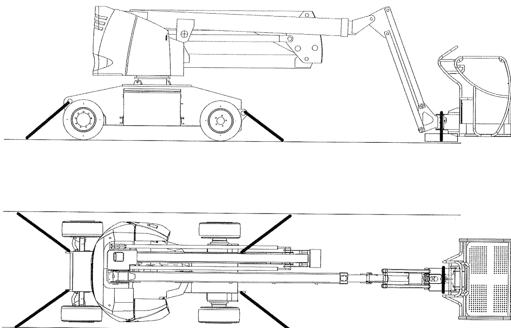
Fig. 8 - Eslingado para transporte
