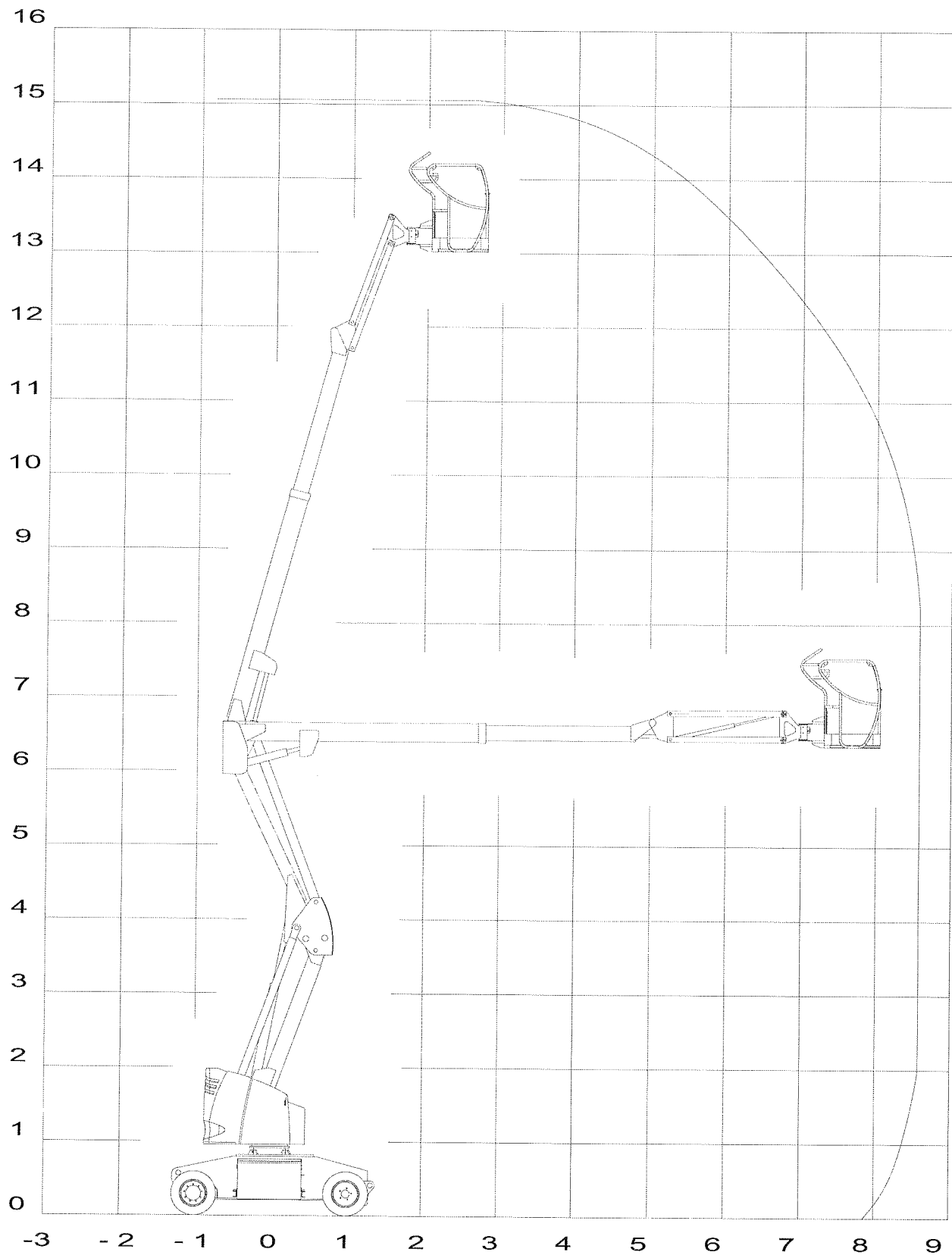
Fig. 3 - Zona de trabajo HA15IP
