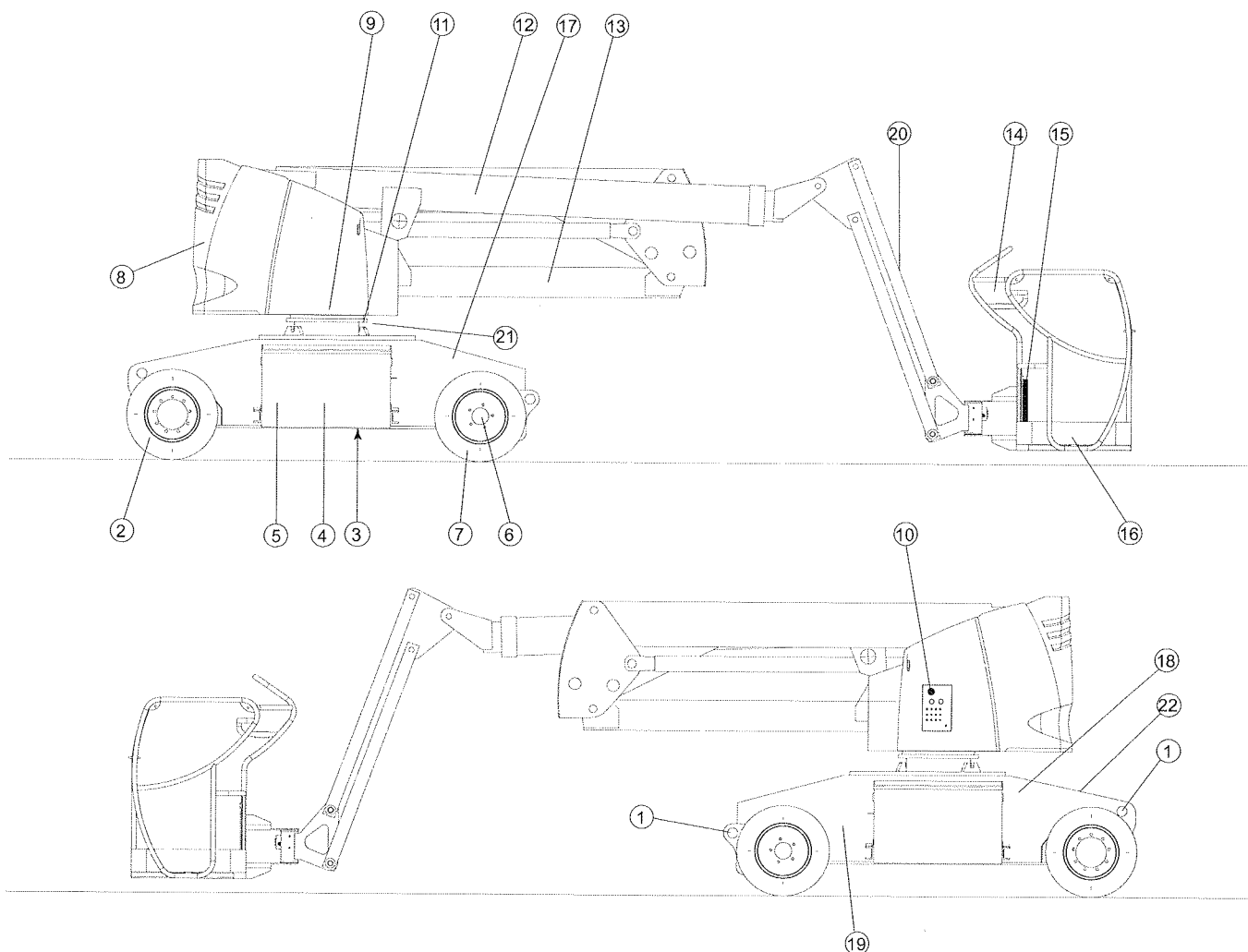
Fig. 2 - Componentes principales
