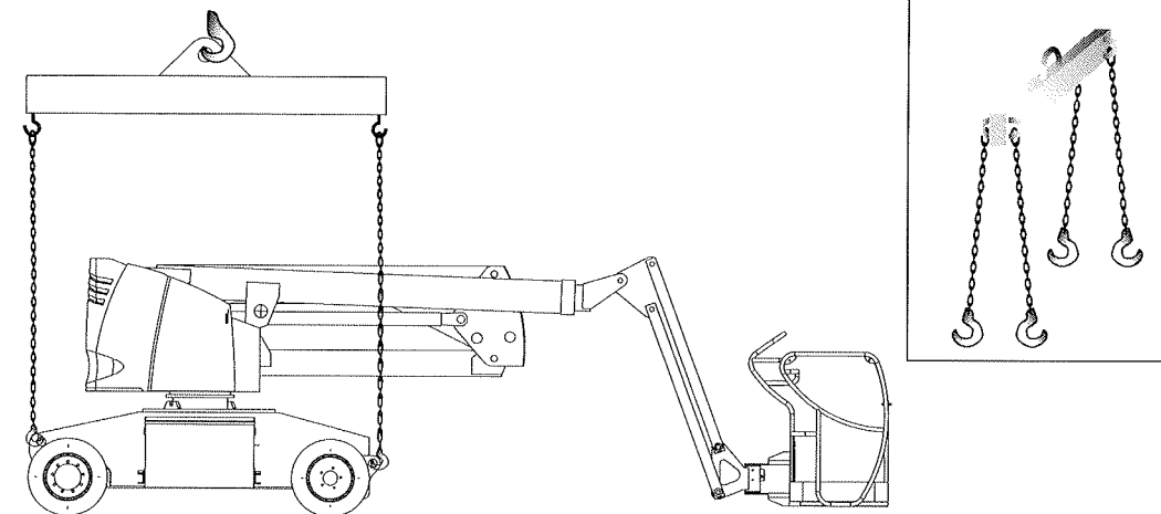
Fig. 6 - Descarga por elevación
